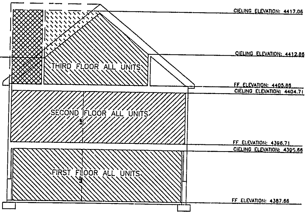
ELEVATION PLAN (BUILDING 6133) SCALE: 1" = 4'-0"
