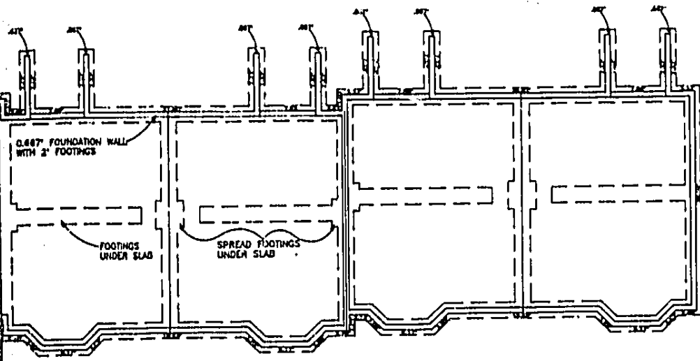
FOUNDATION DING 6133)
