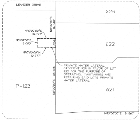
DETAIL "UU" SCALE: 1" = 10'
